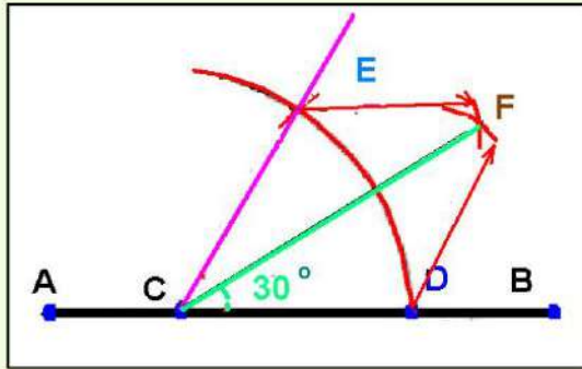
الشكل 11-3 : رسم زاوية قيمتها 30 درجة باستخدام الفرجال.
