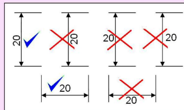
الشكل 29-6 : كتابة قيم الأبعاد.
