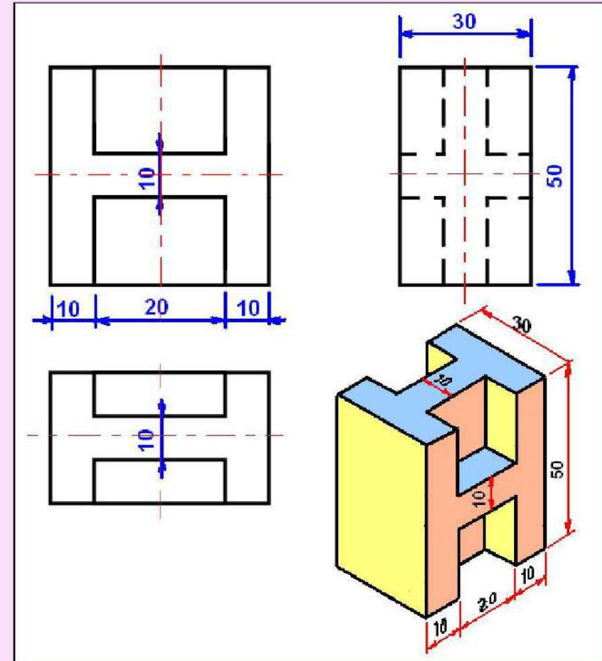
الشكل 47-6 : مساقط لمنظور هندسي متناظر.
