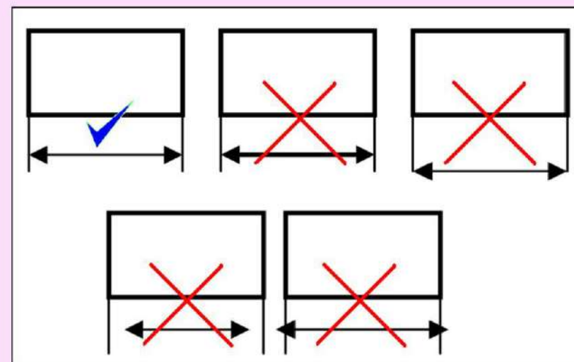
الشكل 28-6 : رسم خط البعد.
