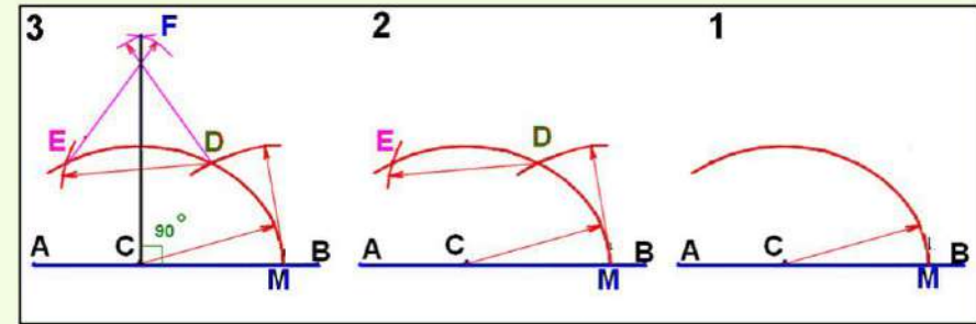
الشكل 3-12 : رسم زاوية قائمة 90 درجة باستخدام الفرجال.
