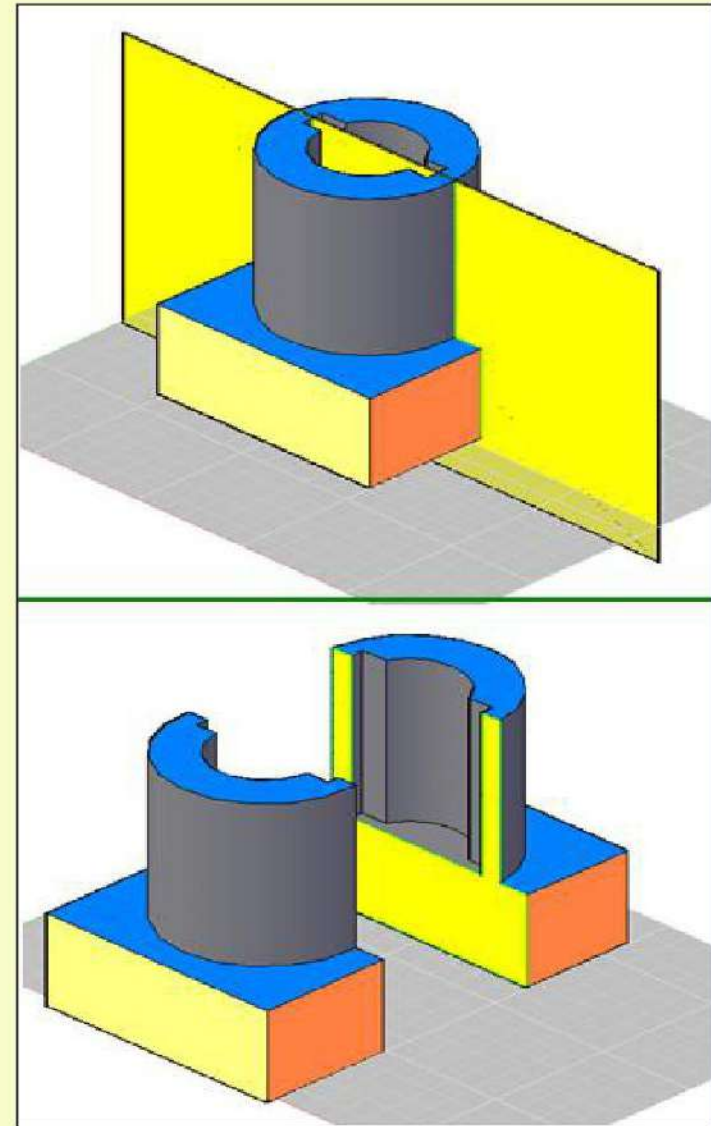
الشكل 20-7 : القطاع الكامل.
