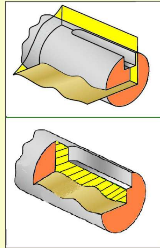
الشكل 24-7 : القطاع الجزئي.
