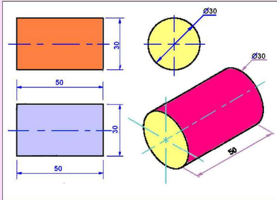
الشكل 38-6 : المساقط الثلاثة لأسطوانة.
