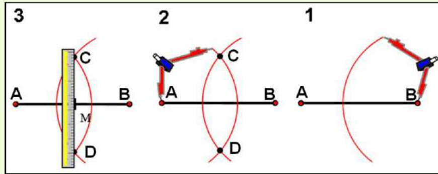
الشكل 2-3 : تصنيف المستقيم باستخدام الفرجال.
