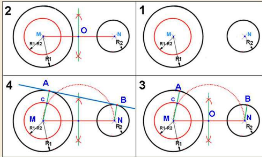
الشكل 4-9 : رسم مماس لدائرتين معلومتين من الخارج.
