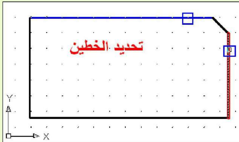
الشكل 9-25 : الشطف (كسر الأركان الحادة).
