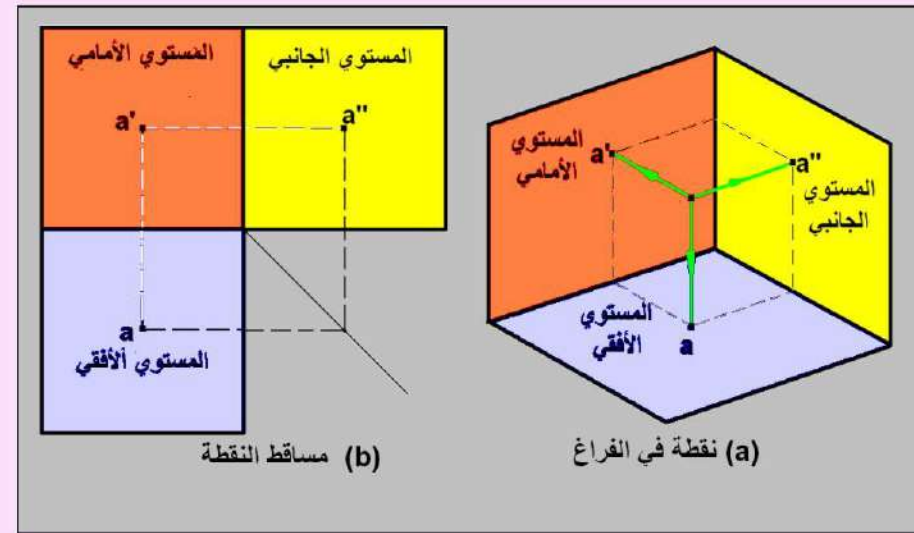
الشكل 12-6 : إسقاط النقطة على مستويات الإسقاط الرئيسية.
