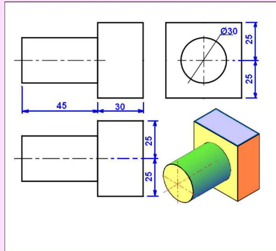
الشكل 6-49 : مساقط لمنظور اسطوانة مثبتة على قاعدة مربعة.
