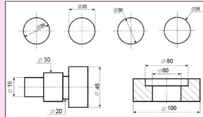
الشكل 32-6 : كتابة أبعاد أقطار الدوائر.
