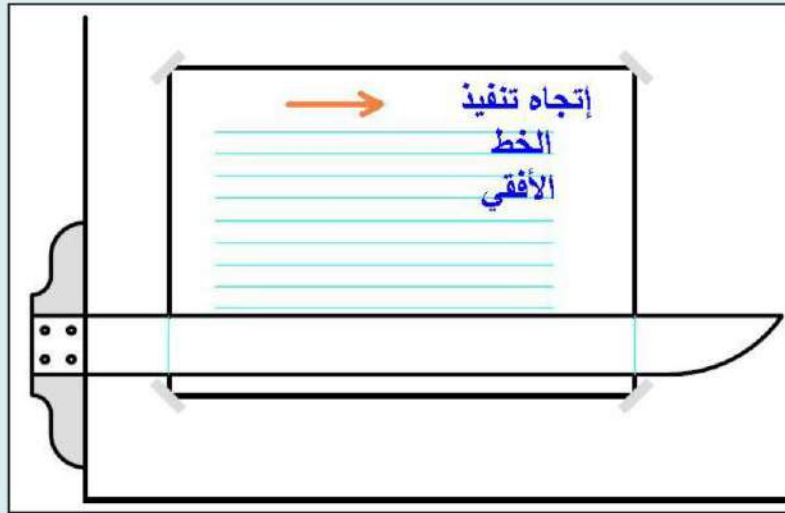
الشكل 3-2 : رسم الخطوط الأفقية بواسطة المسطرة.
