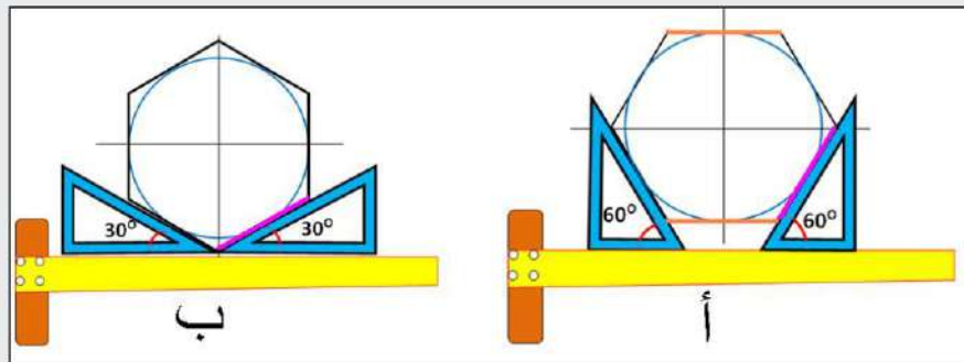
الشكل 11-5 : رسم شكل سداسي باستخدام المثلث.
