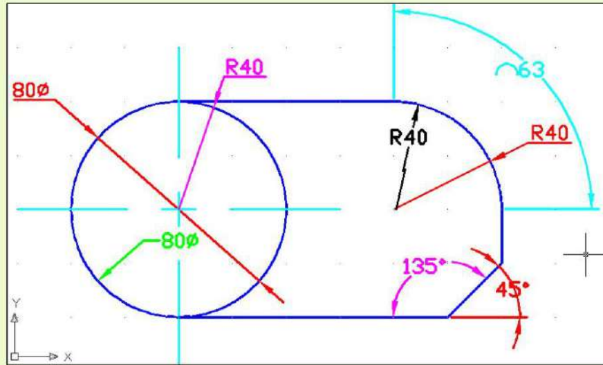
الشكل 9-34 : عدة طرق لوضع أبعاد الدوائر والزوايا.
