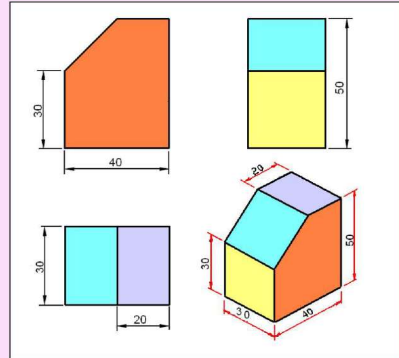
الشكل 37-6 : المساقط الثلاثة لموشور.
