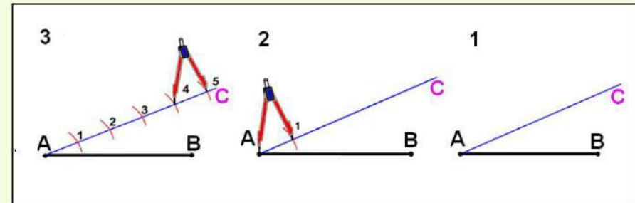
الشكل 3-5 مراحل تقسيم خط مستقيم لخمس أقسام متساوية.
