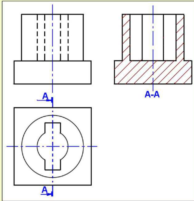
الشكل 21-7 : مقطع جانبي كامل.
