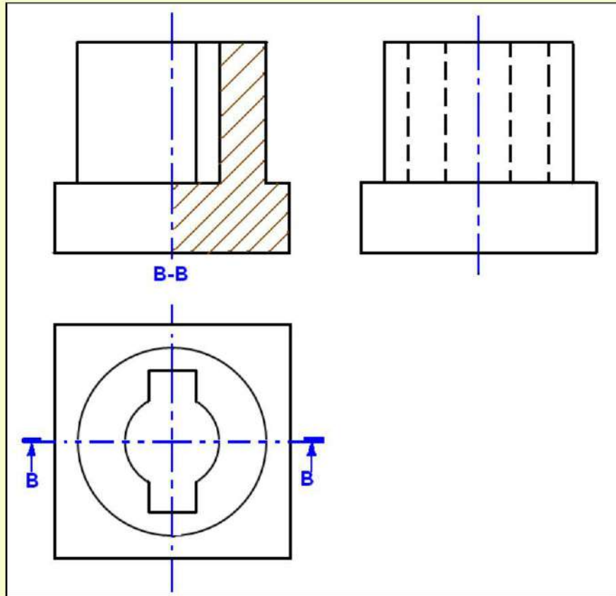
الشكل 7-23 : نصف قطاع أمامي.
