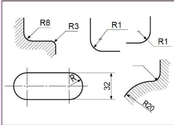
الشكل 33-6 : كتابة أبعاد أنصاف الأقطار.
