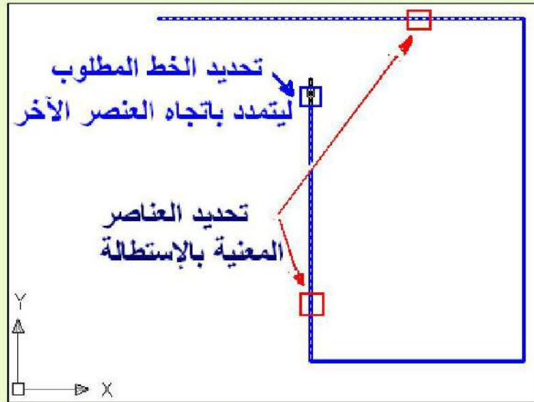
الشكل 24-9: تطويل (مد) خط باتجاه عنصر.
