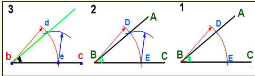
الشكل 14-3: رسم ونقل زاوية ذات قياس معين.
