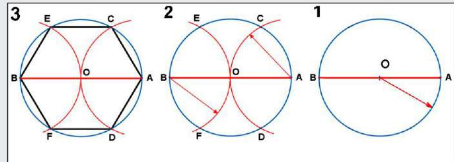
الشكل 10-5 : رسم مضلع سداسي داخل دائرة معلومة.
