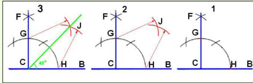
الشكل 3-13 : رسم زاوية قيمتها 45 درجة باستخدام الفرجال.
