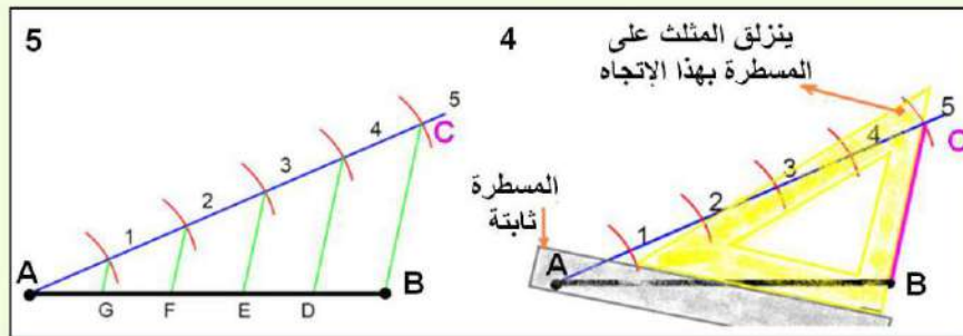
الشكل 3-6 : الحصول على أجزاء متساوية للمستقيم AB.
