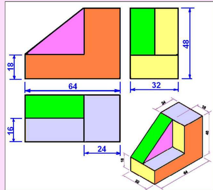
الشكل 41-6 : المساقط الثلاثة لجسم (منظور).
