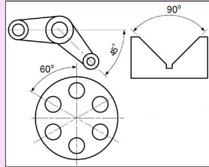
الشكل 31-6 : كتابة قيم الزوايا.
