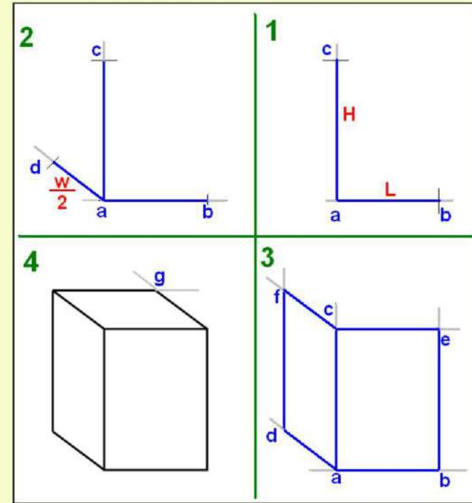
الشكل 13-7 رسم المنظور المائل لمتوازي مستطيلات.
