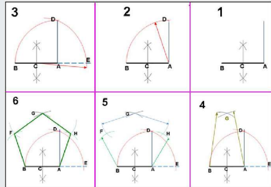
الشكل 5-8 : رسم مخمس بمعلومة طول ضلعه.
