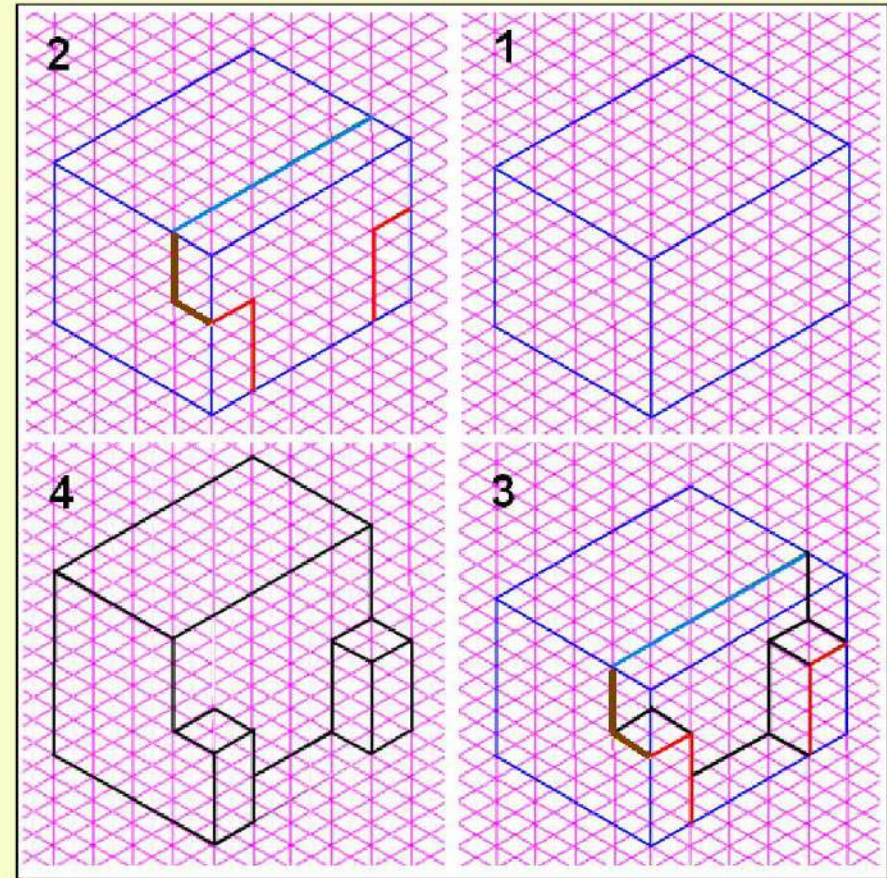
الشكل 7-16 : مراحل رسم منظور أيزومتري على مخطط شبكي.
