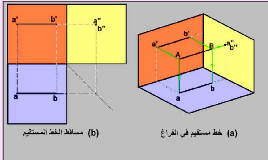
الشكل 13-6 : إسقاط الخط المستقيم على مستويات الإسقاط الرئيسية.
