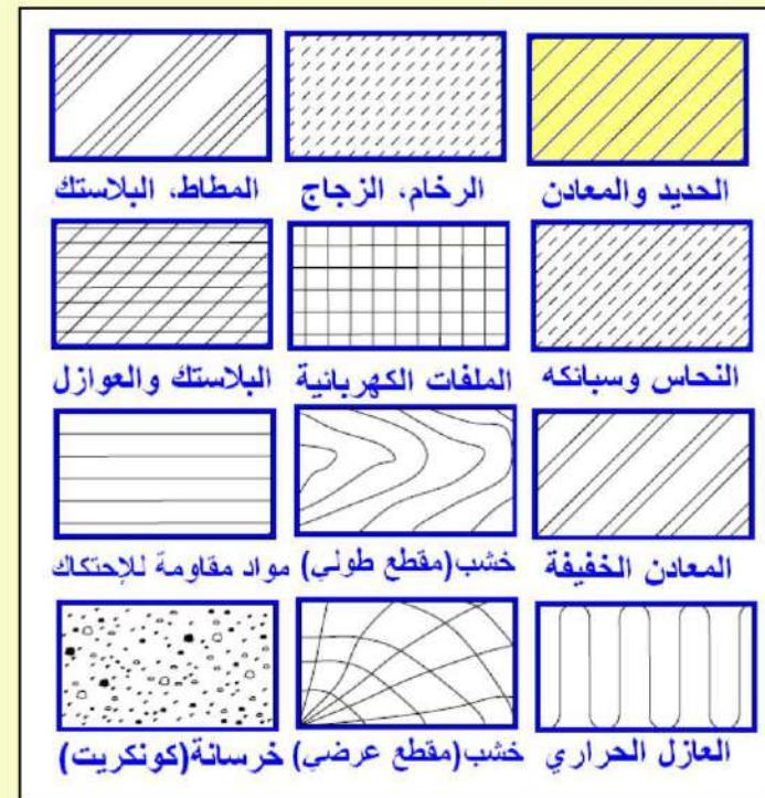
الشكل 19-7 أنواع التهشير حسب نوع المادة.
