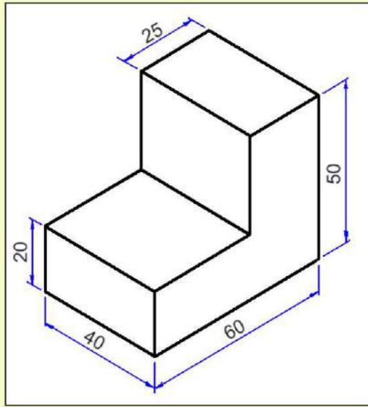
الشكل 7-11 : كتابة الأبعاد على المنظور.
