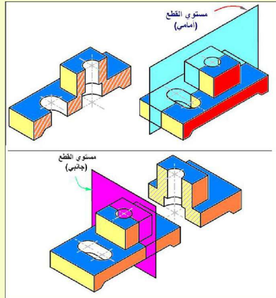
الشكل 7-17: مستويات القطع والأجزاء المقطوعة.
