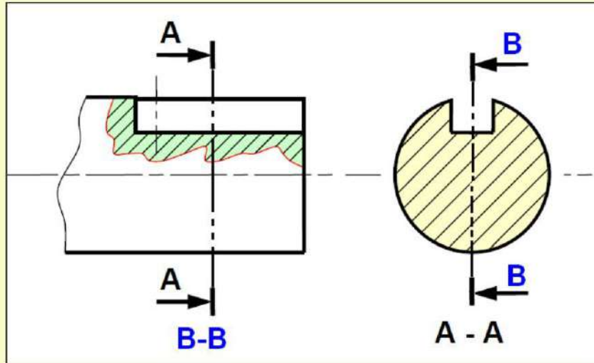
الشكل 25-7 : مسقط أمامي فيه قطاع جزئي.
