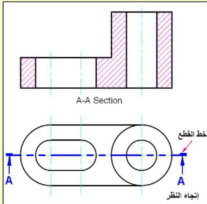
الشكل 7-18: تثبيت خط القطع على المسقط.
