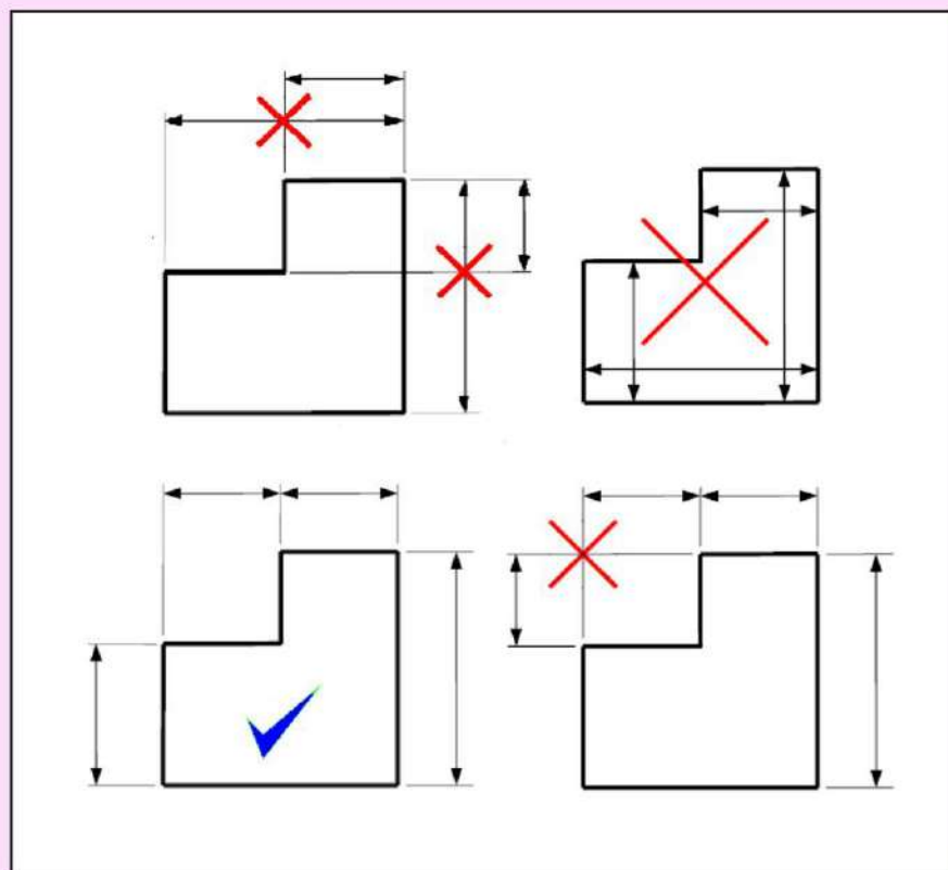
الشكل 30-6 : توزيع الأبعاد على المساقط.
