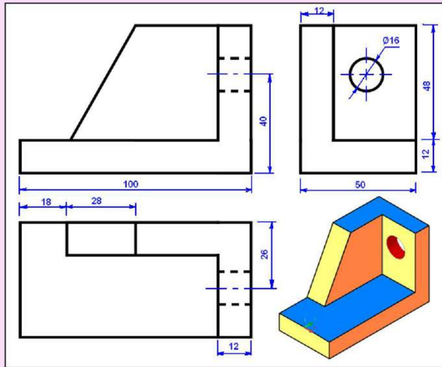
الشكل 6-50 : مساقط لمنظور هندسي يحتوي على سطح مائل.
