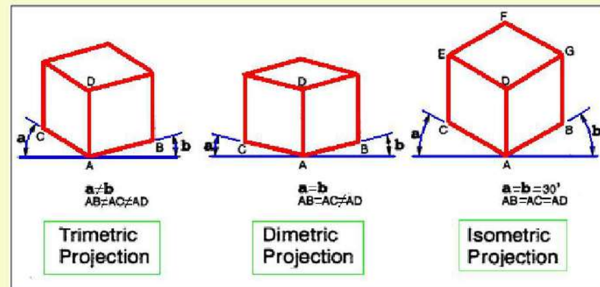
الشكل 2-7 : أنواع الرسم المحوري.
