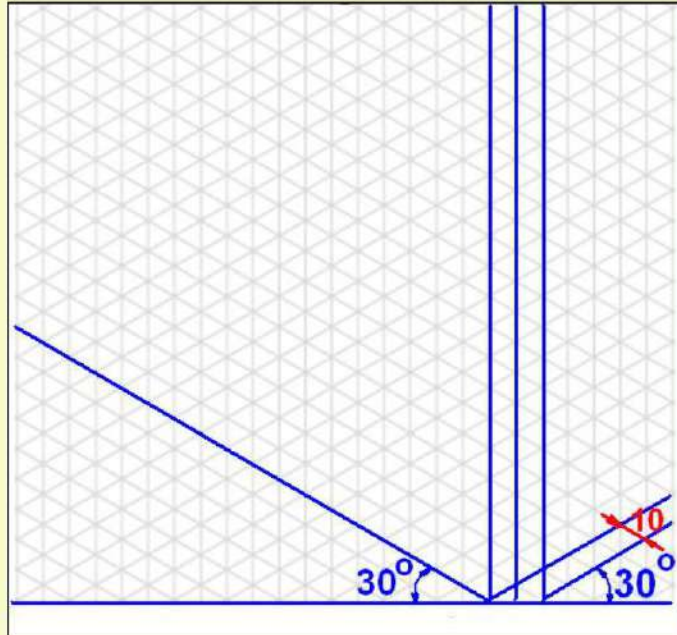
الشكل 14-7 : مخطط شبكي للمنظور الآيزومتري.
