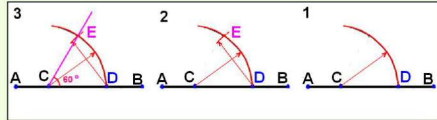
الشكل 10-3 : رسم زاوية قيمتها 60 درجة باستخدام الفرجال.
