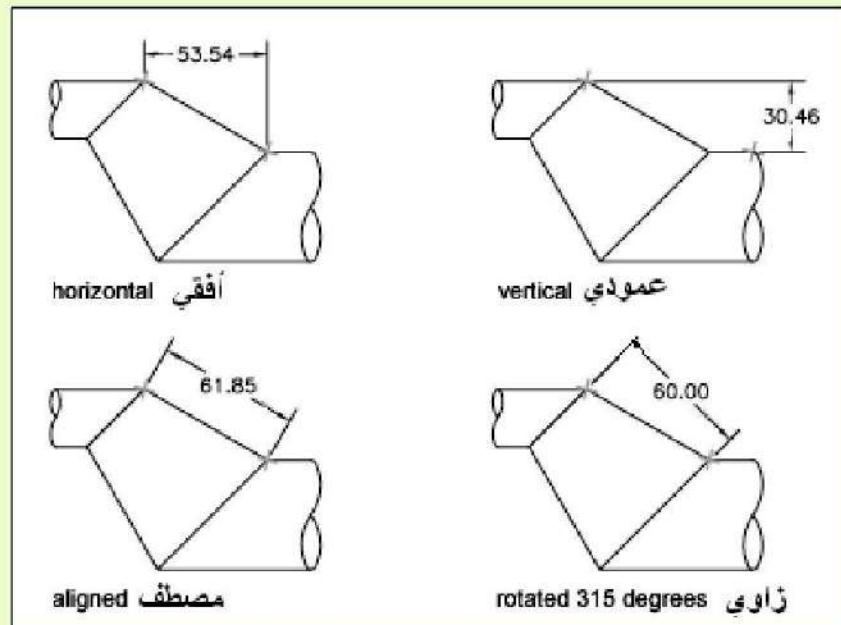
الشكل 9-33 : الأبعاد الخطية.
