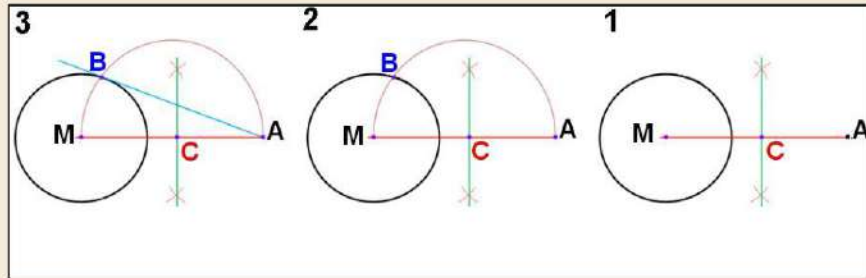
الشكل 5-4 رسم مماس لدائرة من نقطة معلومة خارجة عنها.
