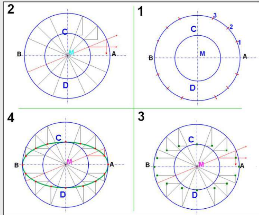
الشكل 14-5 : رسم القطع الناقص بطريقة الدائرتين المتمركزتين.
