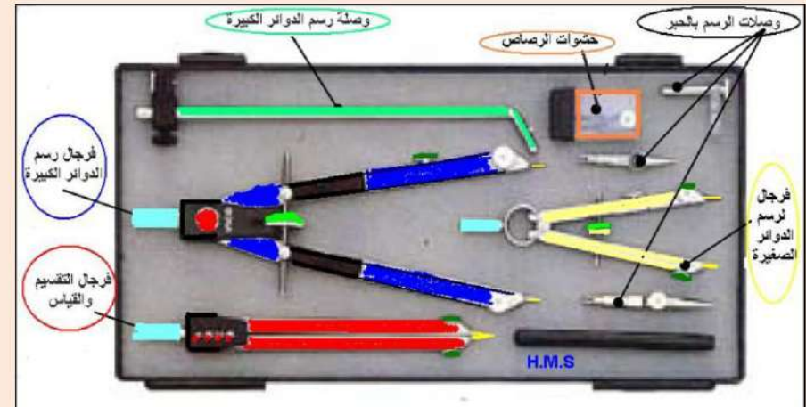
الشكل 5-1 : مجموعة الفرغال والمقسم.
