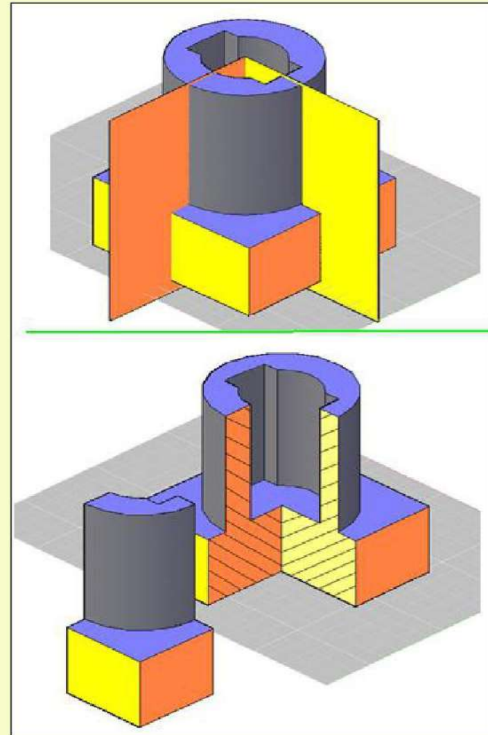
الشكل 7-22 : القطاع النصفى.
