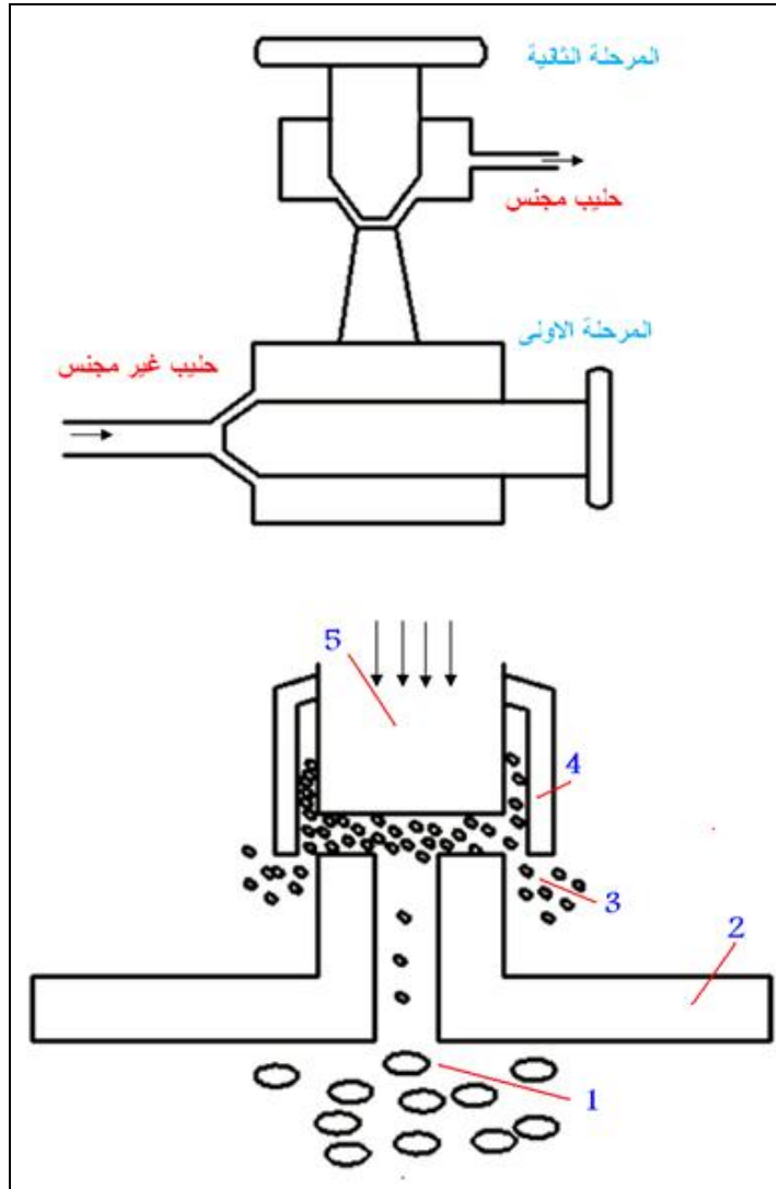
الشكل 8-5 : مراحل عمل مجنس الحليب وصمام التجنيس
