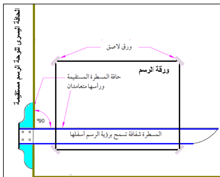
الشكل 1-1: لوحة الرسم مع مسطرة T
