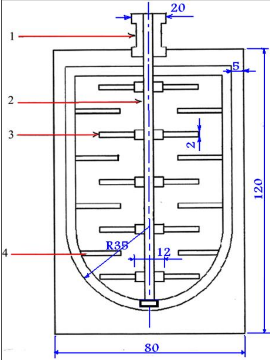
الشكل 5-7 : مخطط لخلاط ذي الحركة المزدوجة
