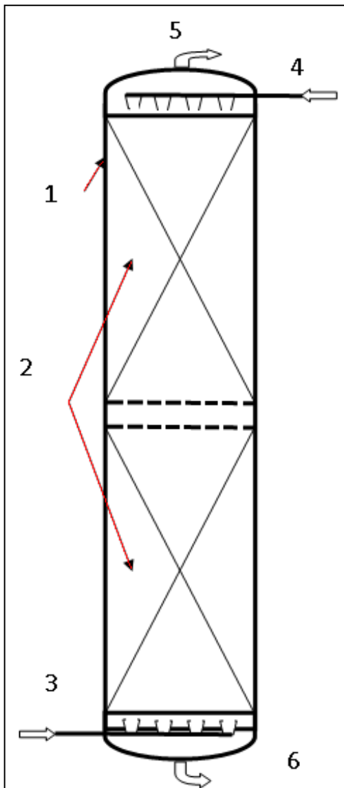
الشكل 2-5: مخطط مقطع طولي لبرج الامتصاص ذي الحشوة
