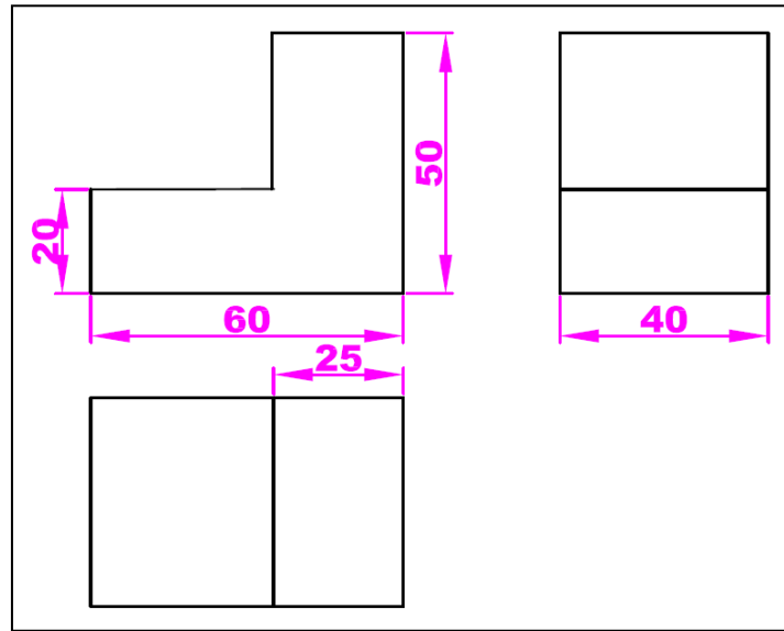
الشكل 3-7: المساقط الثلاثة لمنظور
