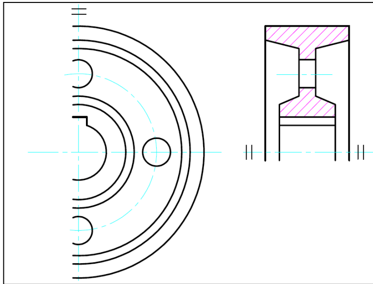
الشكل 14-2: القطاع المتماثل
