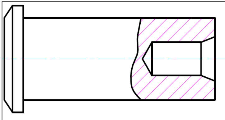
شكل 2-8: القطاع الجزئي
