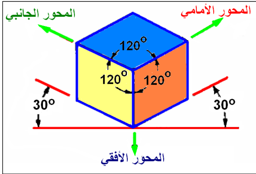
الشكل 3-5 : طريقة رسم المنظور الأيزومتري
