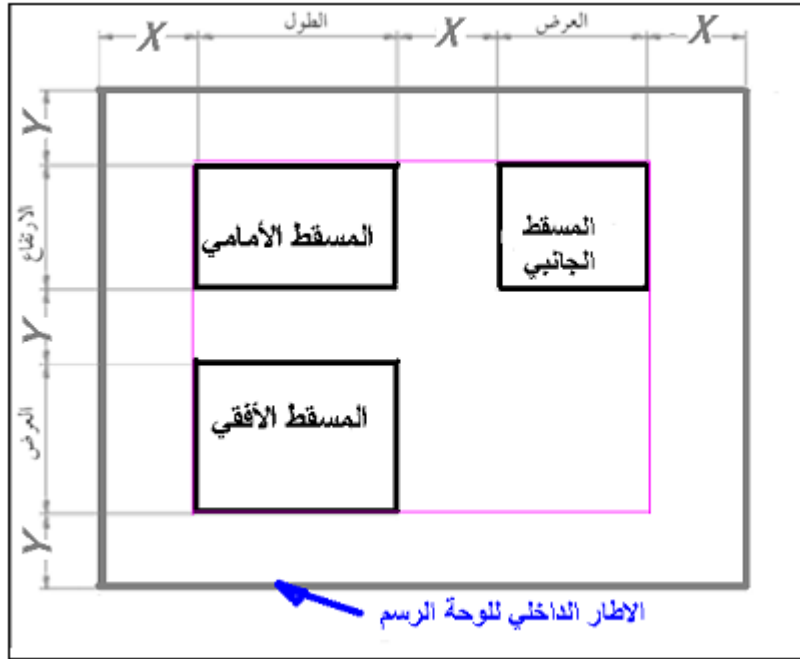
الشكل 8-1: توزيع المساقط على ورقة الرسم
