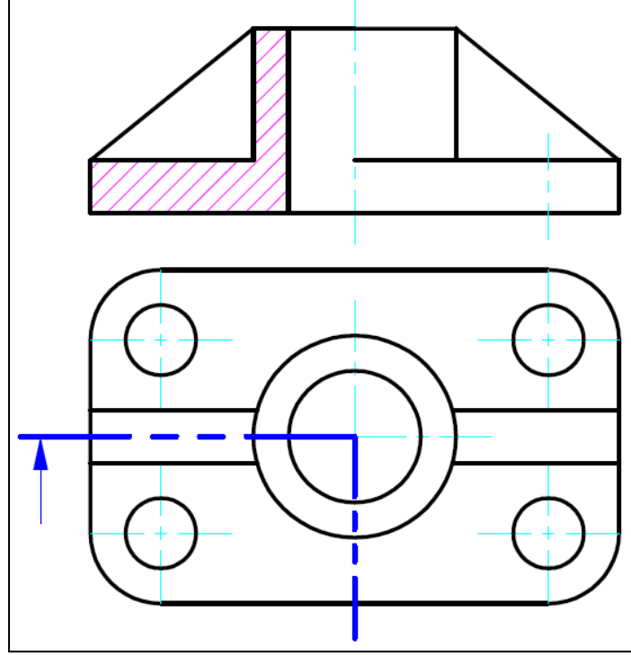
الشكل 2-7: نصف القطاع
