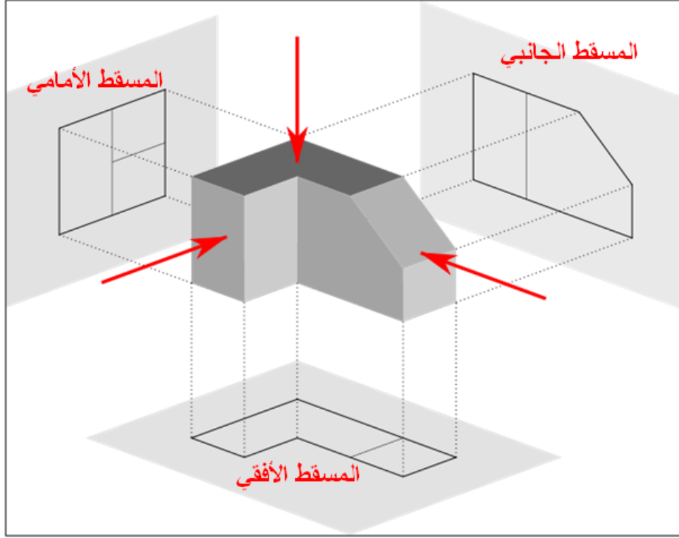
الشكل 6-1 : المنظور ومساقطه المتعامدة
