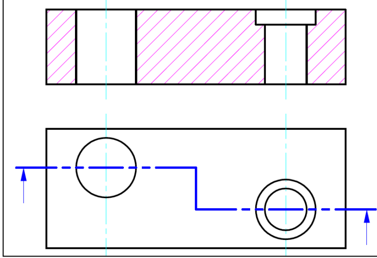
الشكل 11-2: قطاع الإزاحة
