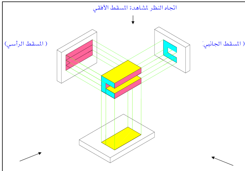
الشكل 1-3: الإسقاط العمودي
