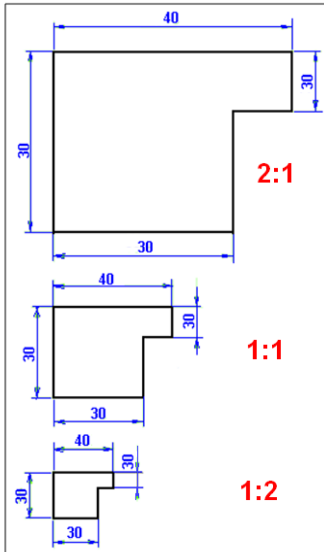
الشكل 5-1 : مقياس الرسم التكبير والتصغير والكامل
