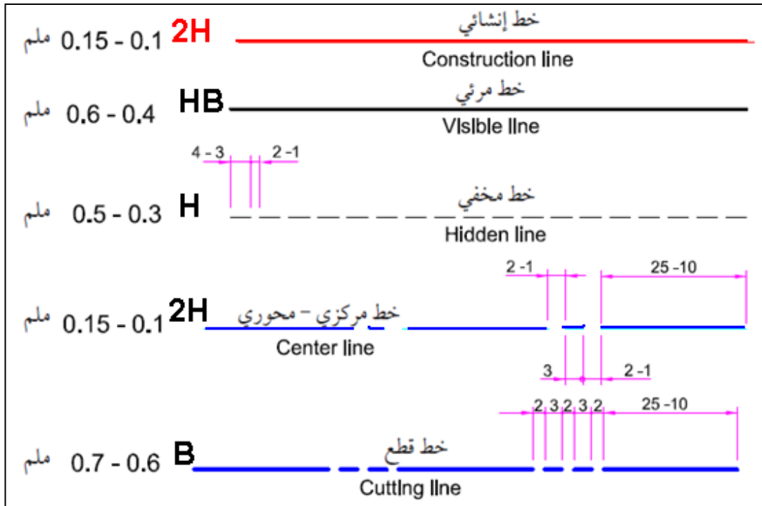
الشكل 3-1: أنواع الخطوط وخواصها
