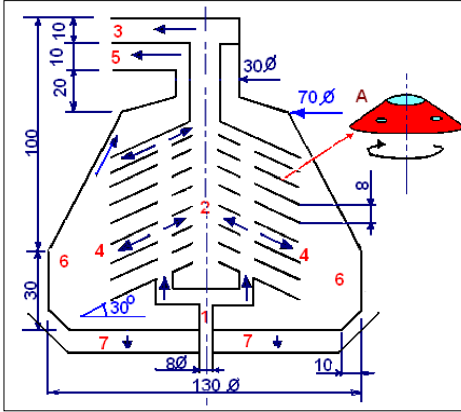
(A) القرص المخروطي (منظور) وتظهر فيه قنوات توزيع الحليب ليدور داخل الفراز:
