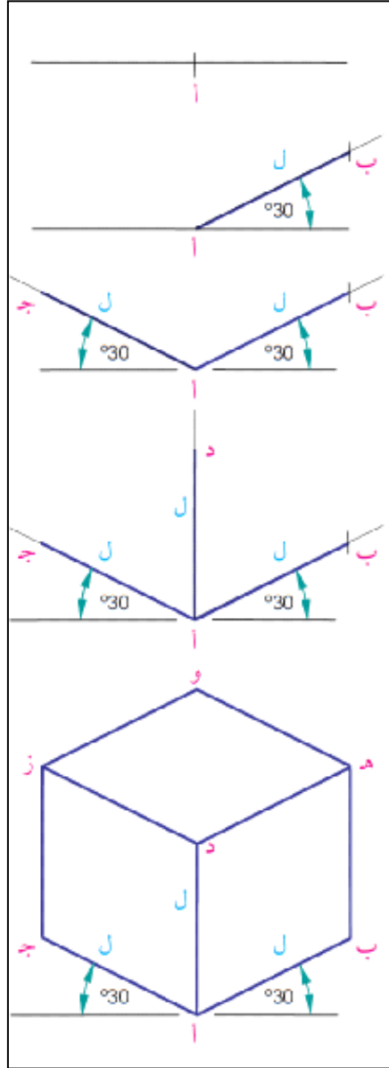
الشكل 3-6: طريقة رسم مكعب
