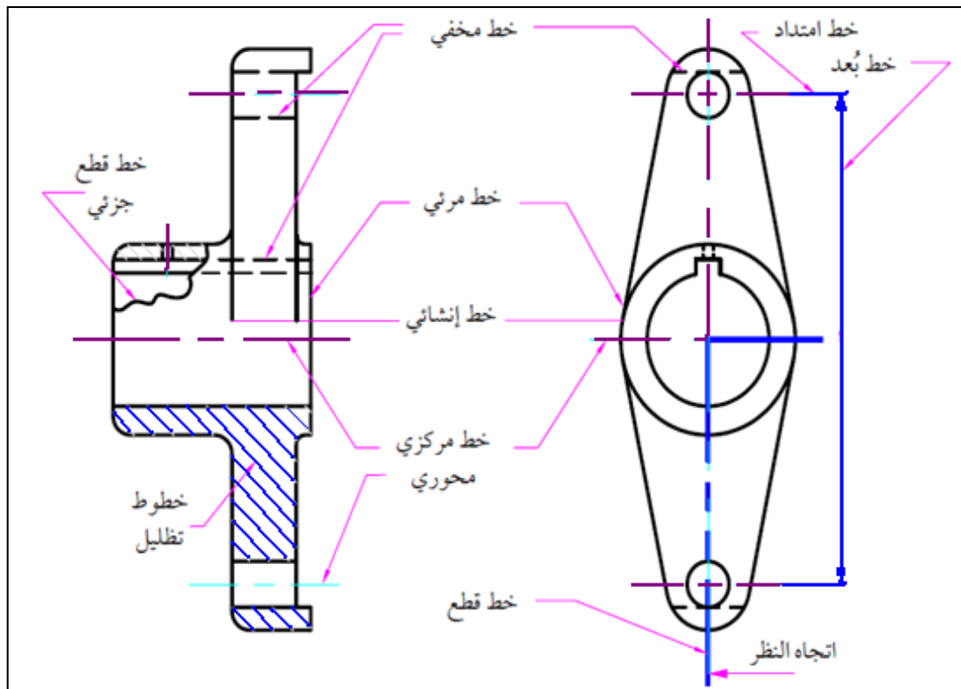
الشكل 4-1: مقطع نصفى أمامي ومسقط جانبي يبين أنواع الخطوط
