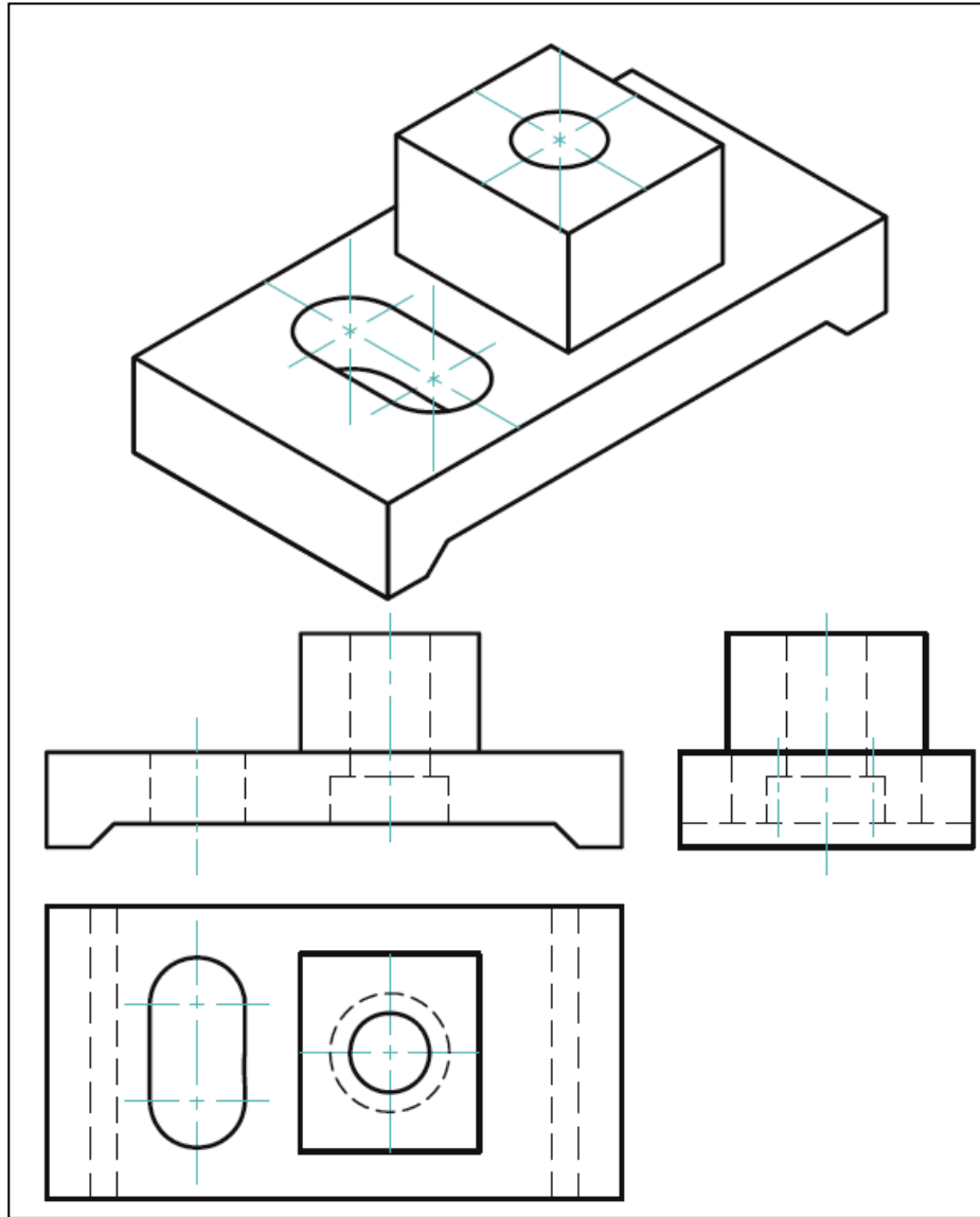
الشكل 1-2 : منظور ومساقطه الثلاثة (لاحظ تشابك الخطوط المخفية)
