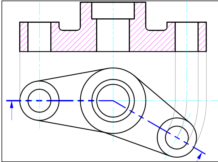
الشكل 12-2: قطاع المحاذاة
