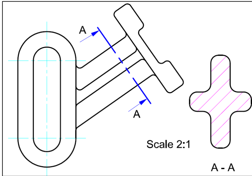
الشكل 10-2: القطاع المنقول
