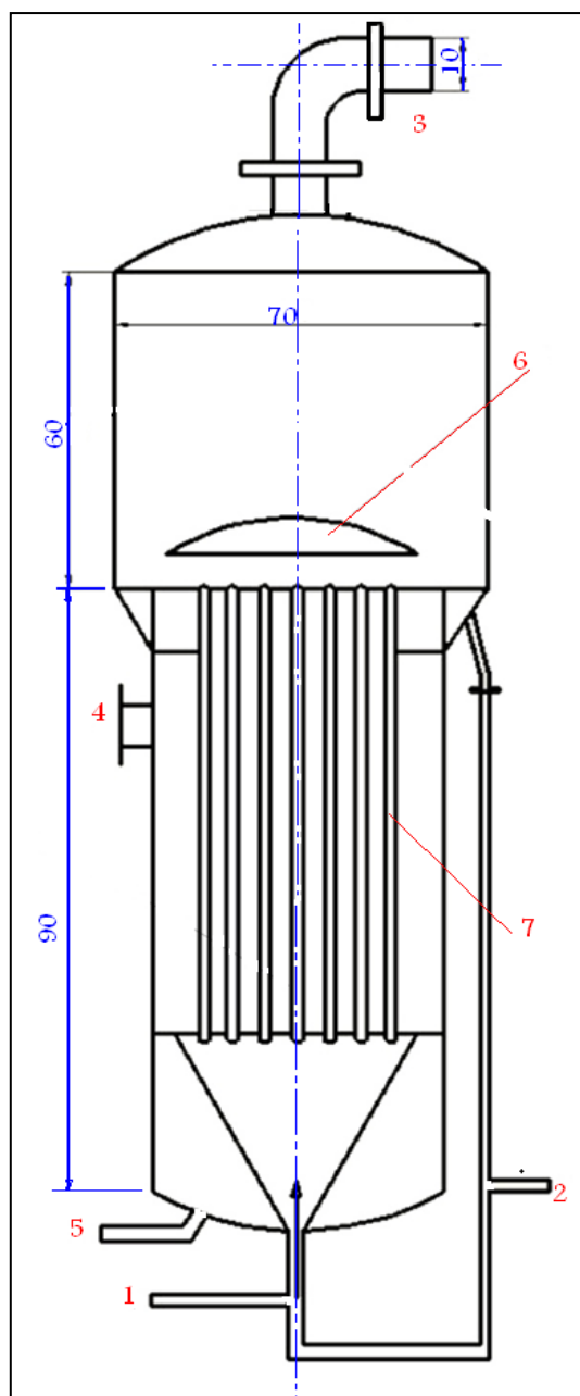
الشكل 5-5 : مخطط لمقطع طولى لمبخرة ذات أنابيب عمودية
