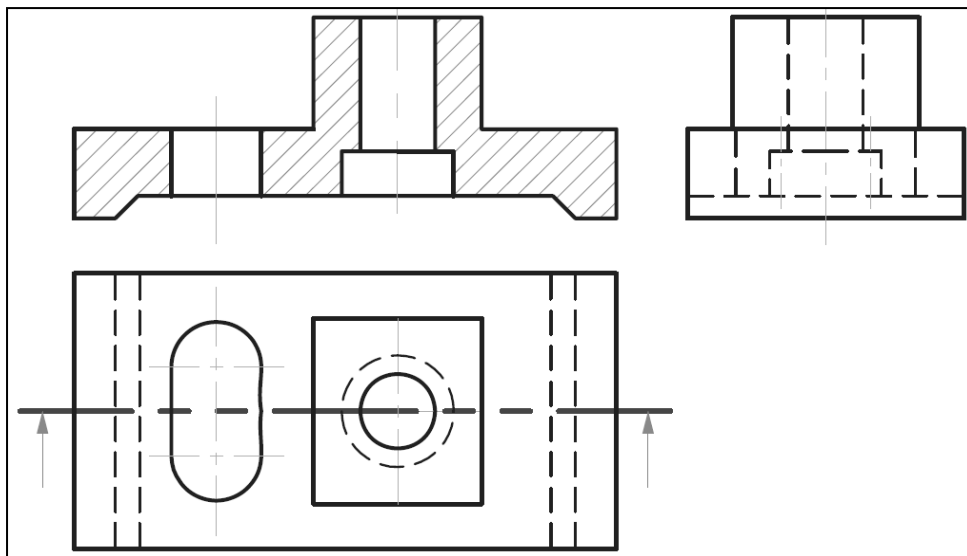
الشكل 2-3 : قطاع أمامي مع بقية المساقط
