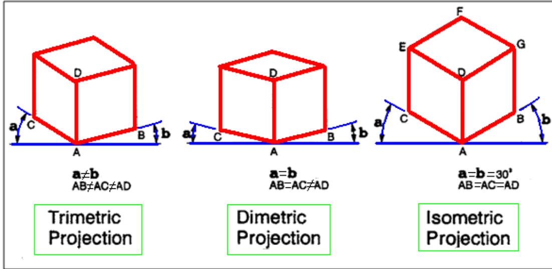
الشكل 3-3 : أنواع الإسقاط المتقايس
