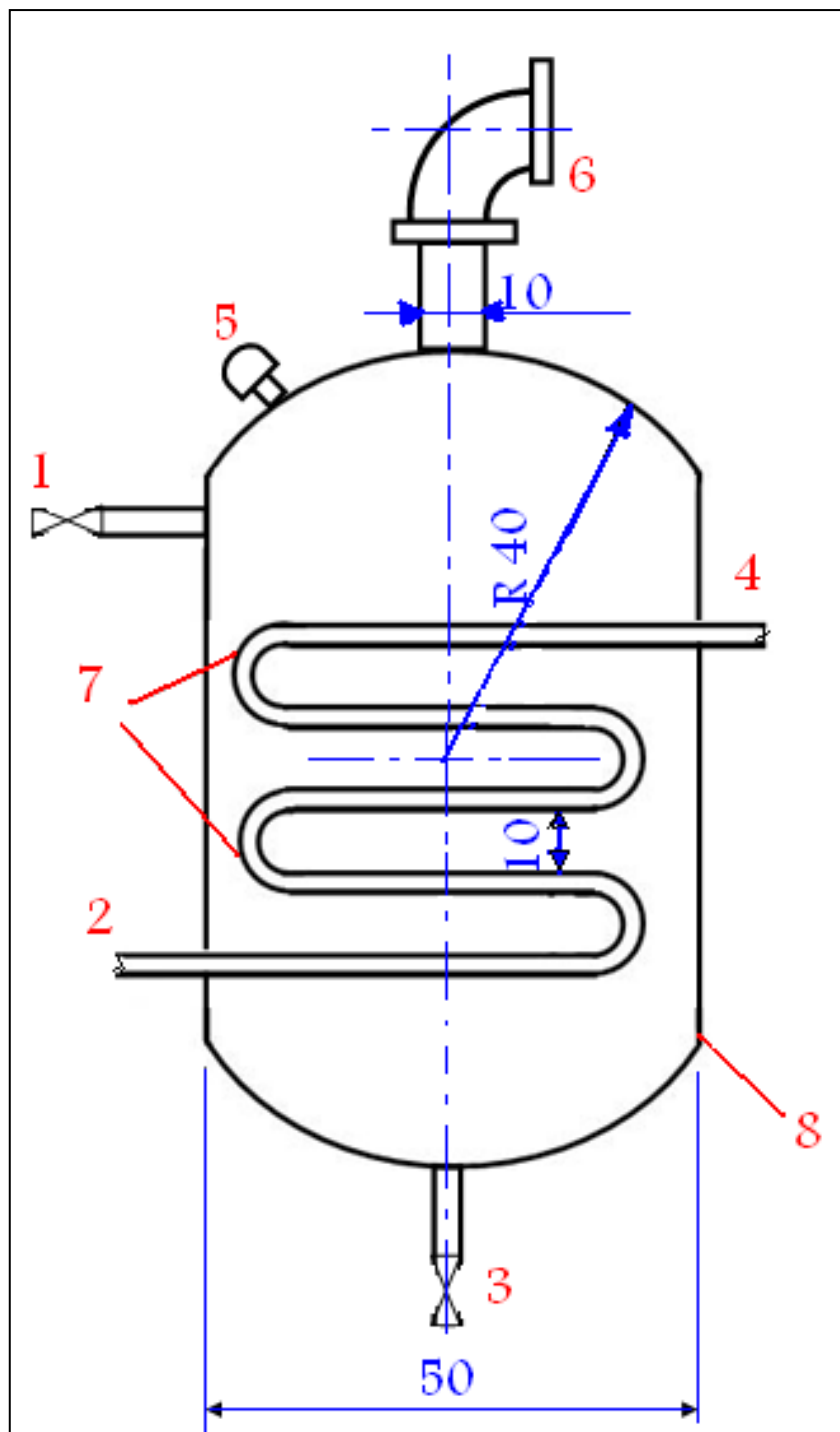
الشكل 4-5 : مخطط لمقطع طولي لمبخرة ذات أنابيب أفقية
