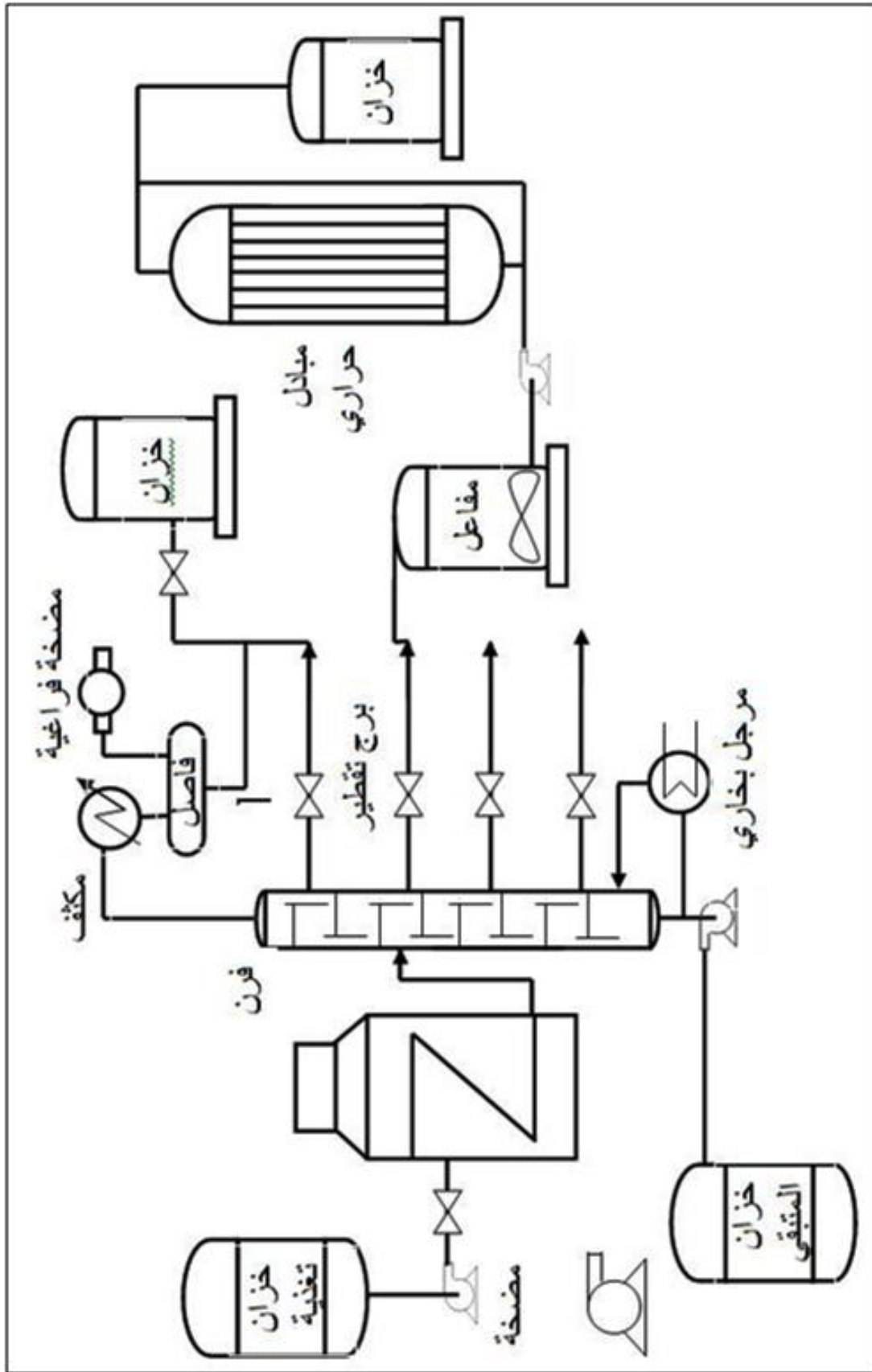
الشكل (1-4) أنموذج يبين ربط الأجهزة في العمليات الصناعية.
