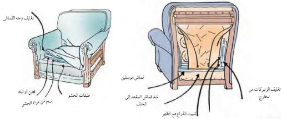
شكل (4-45) يوضح كيفية تنجيد القاعدة والظهر
