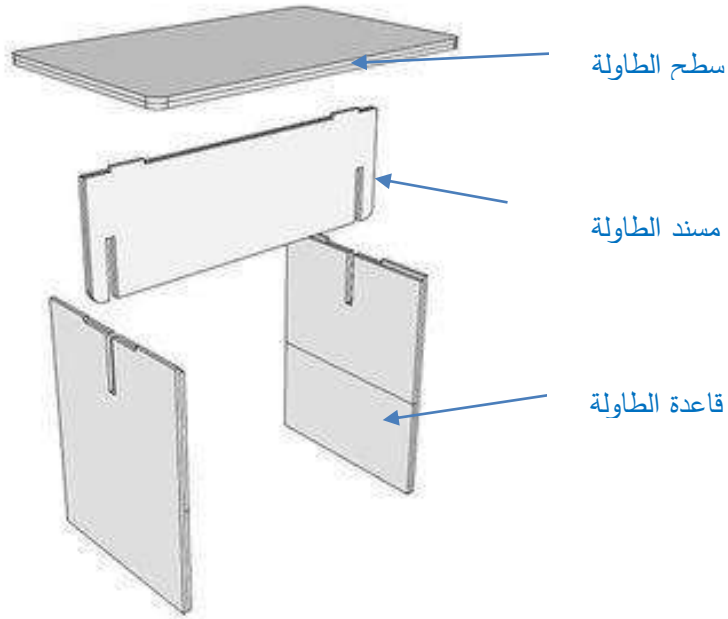
الشكل (5-26) يوضح تشكيل طاوله بواسطه التعشيق
