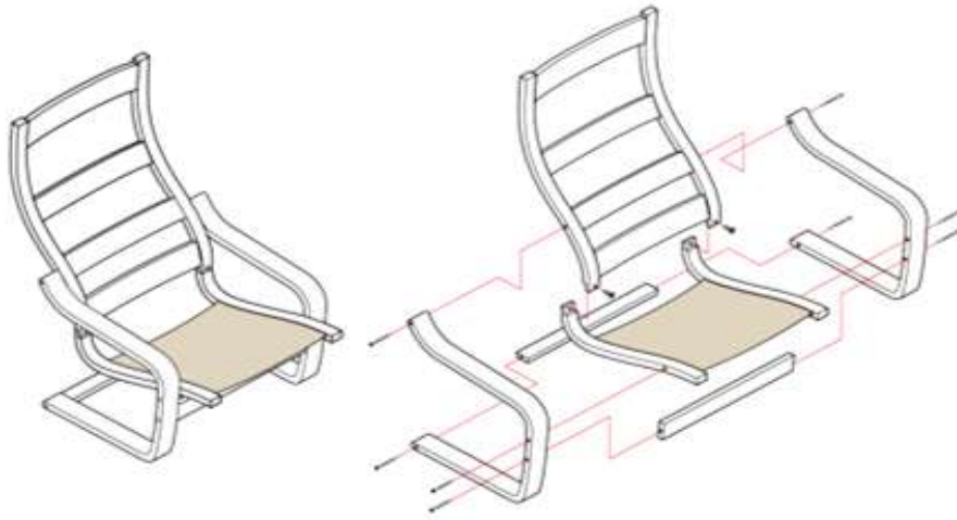
شكل (3-18) يوضح طبيعة الرسم التجميعي لإيضاح كيفية ارتباط أجزاء الأثاث مع بعضها الآخر
