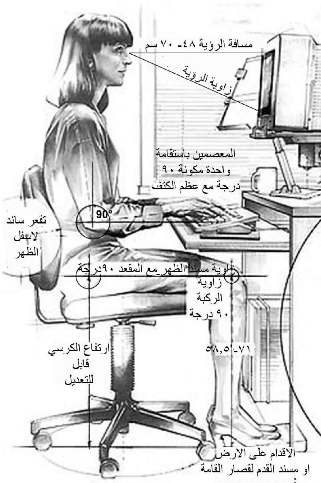
شكل (3-2) الحسابات القياسية المثالية لتصميم الكرسي
