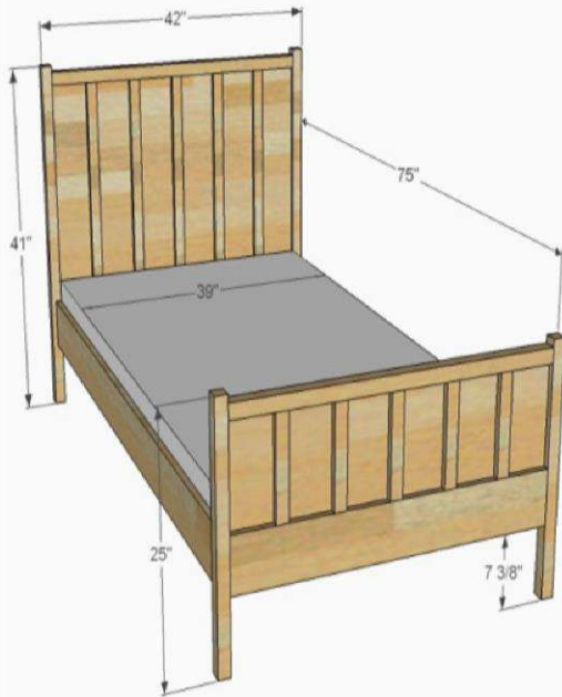
المخطط (5-6) الأبعاد القياسية لسرير لفرد واحد
