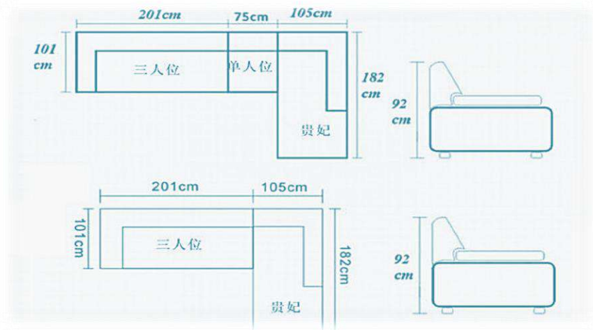
شكل (22-6) الأبعاد القياسية لنوعين من الكنبات القطاعية
