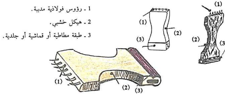
شكل (4-26) مشد الأقمشة الخاص بالتنجيد
