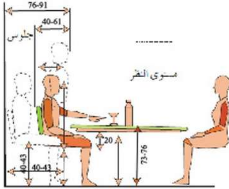
شكل (15-2) الأبعاد القياسية لمنضدة طعام دائرية والكراسي الخاصة بها وكيفية حساب الأبعاد المكانية للكراسي والمنضدة والمساحات الضرورية للحركة والتنقل
