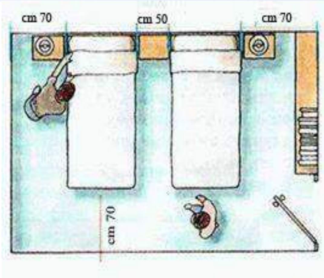
شكل (2-17) مكونات غرفة نوم لفردين وكيفية تنظيم الأسرة بحجومها ووحداتها التكميلية مع المساحة الكلية للفضاء بما يتيح إمكانية وضع مساحة كافية للحركة والتنقل
