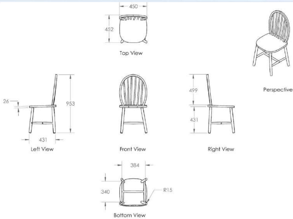
شكل (3-17) يوضح طبيعة الاظهار القياسي للثلاث لبيان الجوانب الأساسية للثلاث والمقاسات والوجه
