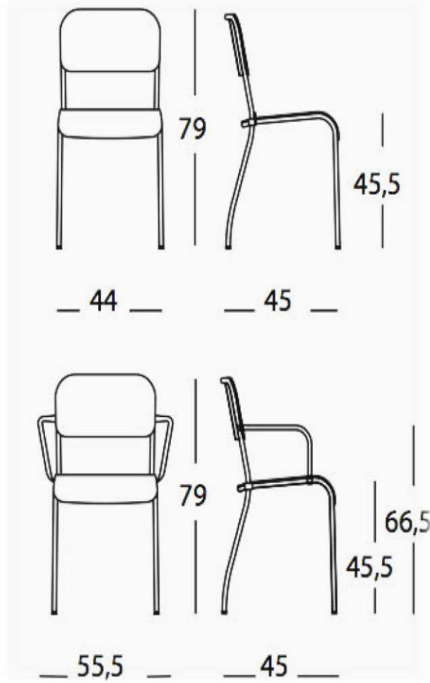
شكل(12-6) الابعاد القياسية لكرسي جلوس بمسند ومن دون مسند
