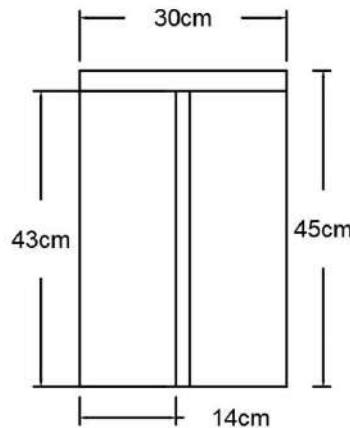
الشكل (5-32) يوضح تركيب الستول باللدائن مع الخشب
