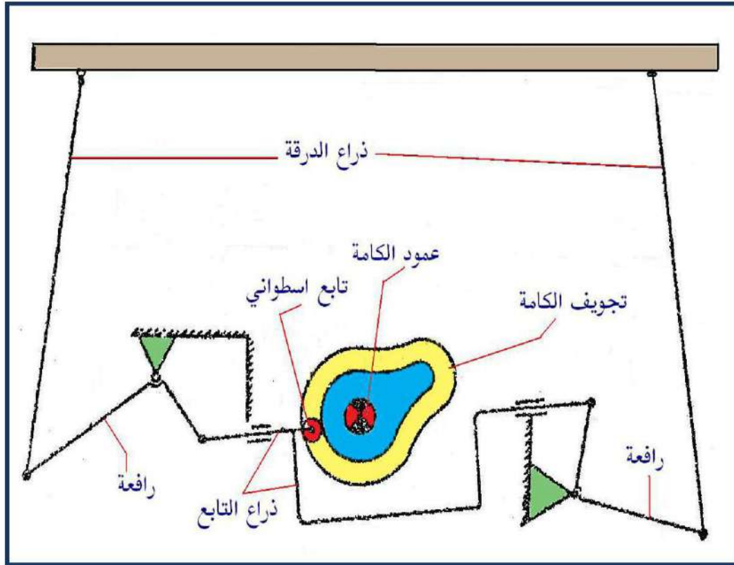
الشكل رقم ( 10-1 ). يبين جهاز الكامات الموجبة الداخلية
