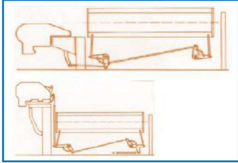
الشكل رقم ( 18 - 1 ) يبين اتصال الدرقات في جهاز الدوبي السالب
