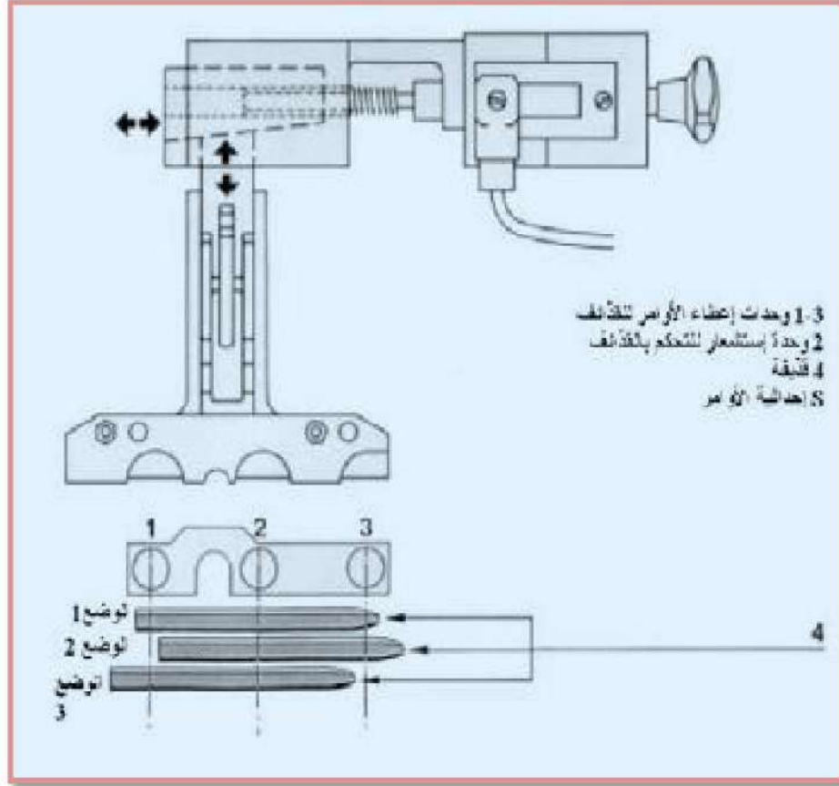
الشكل رقم ( 12-2 ) جهاز الإيقاف الإلكتروني
